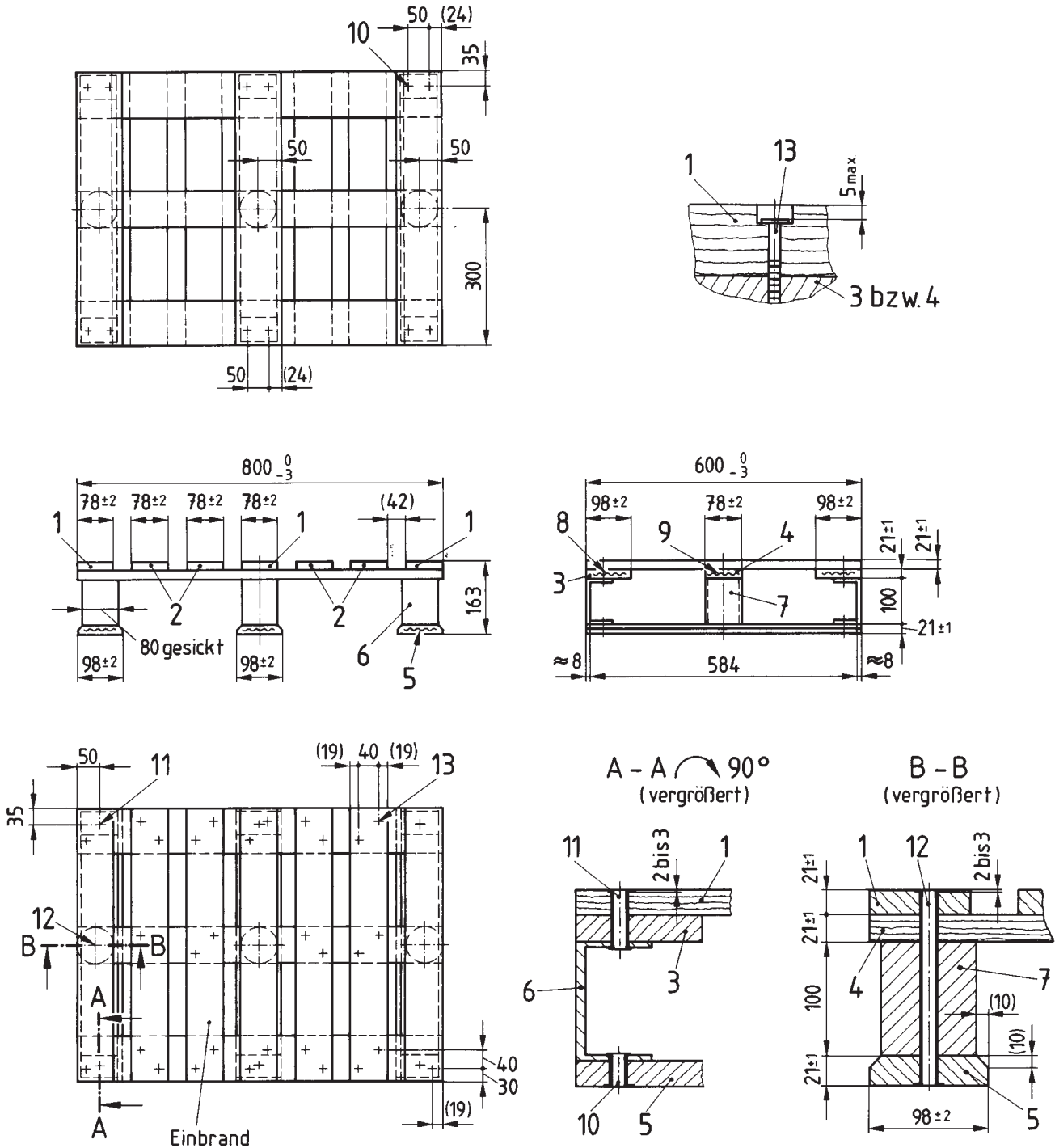
Bild 1. Vierwege-Flachpalette 800 mm × 600 mm
